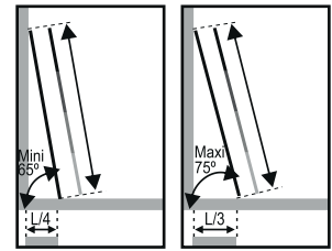
Grado de inclinación en uso 65°-75°
