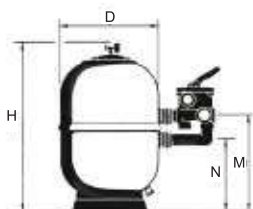
Medidas (mm) DØ=500 / H=770 / M=415 / N=290.
