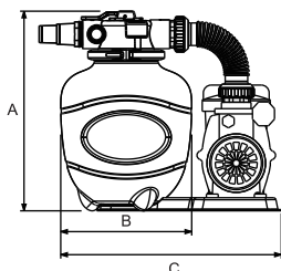
Medidas (mm) A=380 / B=250 / C=430.
